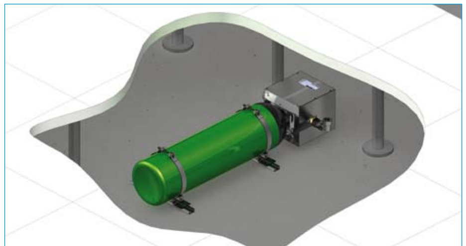
Löschmittelbehälter im Doppelboden (mit Ventil- und Schutzhaube)
